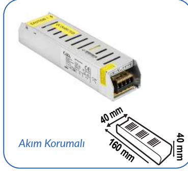
24V 5A 120W SLIM KASA TRAFO
