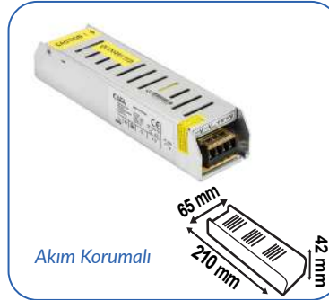
12V 30A 360W SLIM KASA TRAFO
