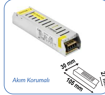
12V 5A 60W SLIM KASA TRAFO
