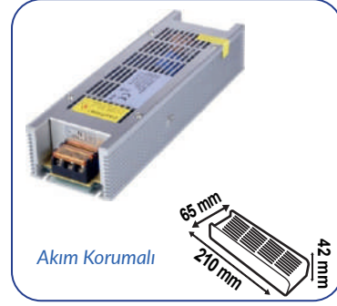
24V 20A 500W SLIM KASA TRAFO
