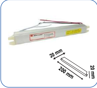
12V 3A 36W KALEM TİPİ TRAF0
