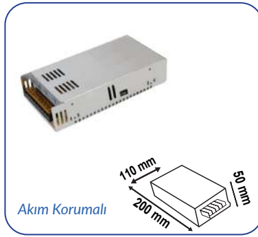
5V 40A 200W KALIN KASA TRAFİ
