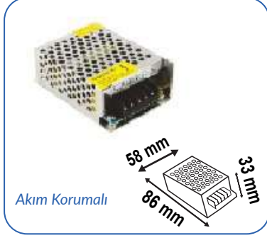
24V 2A 48W KALIN KASA TRAFİ
