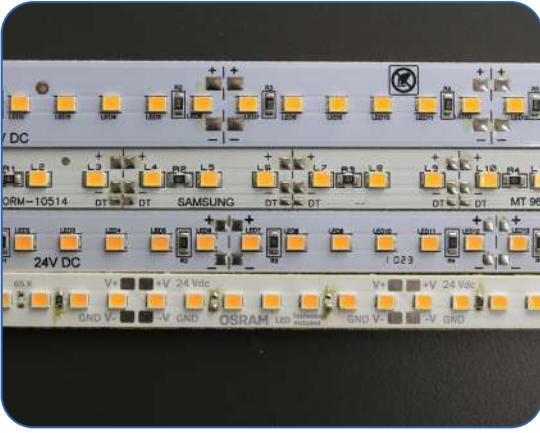
Çubuk (PCB) Led Dizgi Çeşitleri
