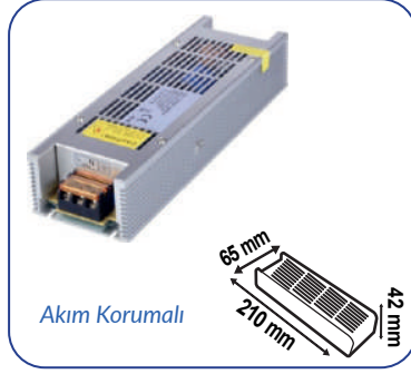
24V 15A 360W SLIM KASA TRAFO
