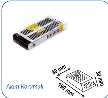
5V 40A 200W SLİM KASA TRAFİ
