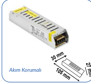
12V 3A 36W SLIM KASA TRAFO
