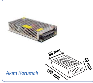
24V 3A 72W KALIN KASA TRAFİ
