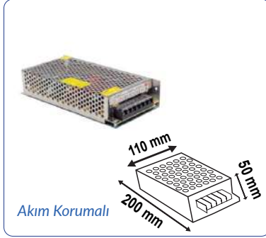
24V 10A 240W KALIN KASA TRAFİ
