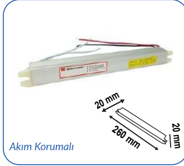
12V 5A 60W KALEM TİPİ TRAF0
