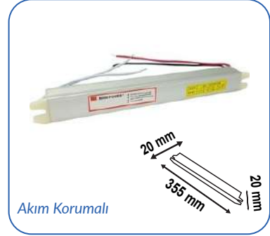
12V 6A 72W KALEM TİPİ TRAF0
