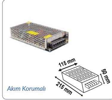
24V 15A 360W KALIN KASA TRAFİ
