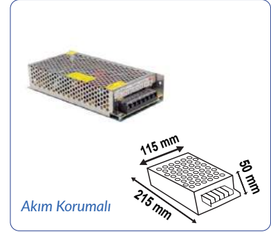
24V 20A 500W KALIN KASA TRAFİ
