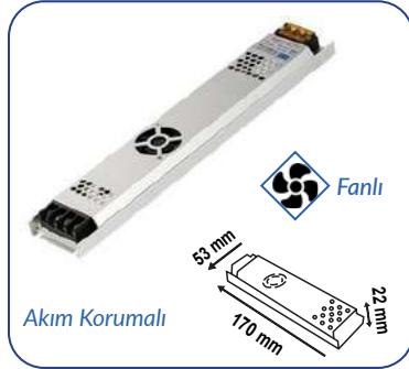
12V 10A 120W ULTRA SLİM TRAF0
