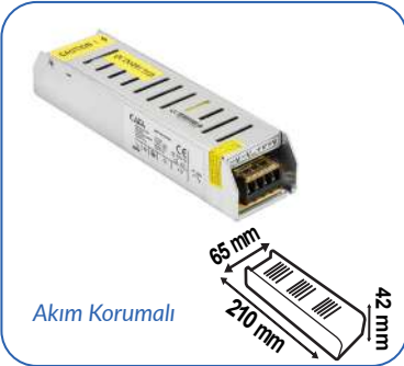
12V 20A 250W SLIM KASA TRAFO
