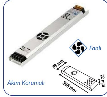
12V 25A 300W ULTRA SLİM TRAF0
